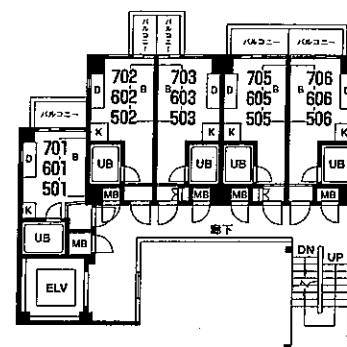
<5・6・7階平面図>
