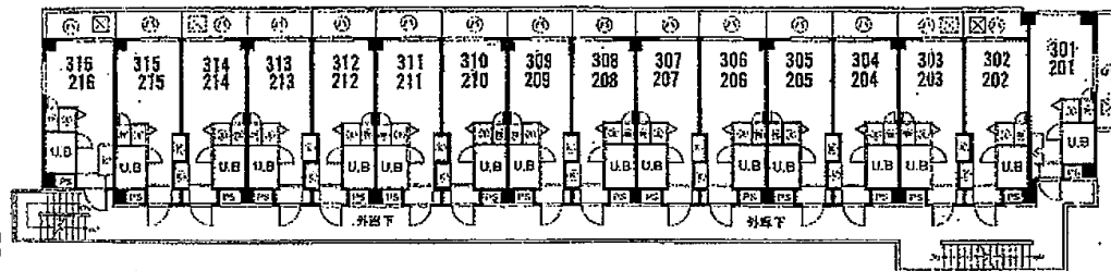
▲2.3階平面図
