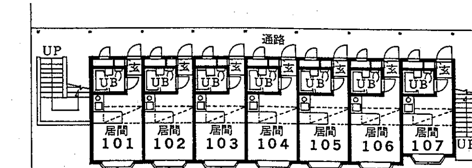
1階平面図
