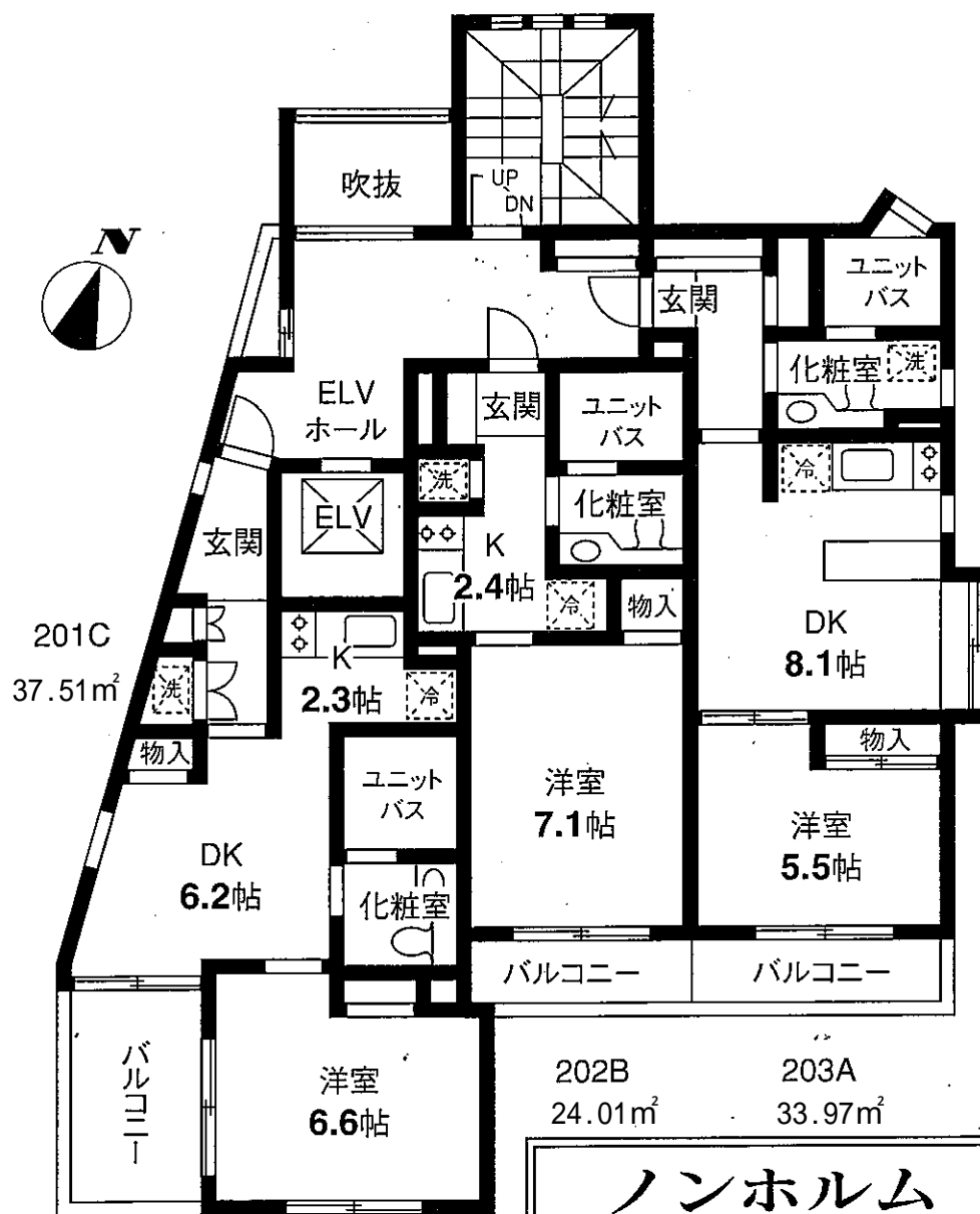
《2階平面図》
