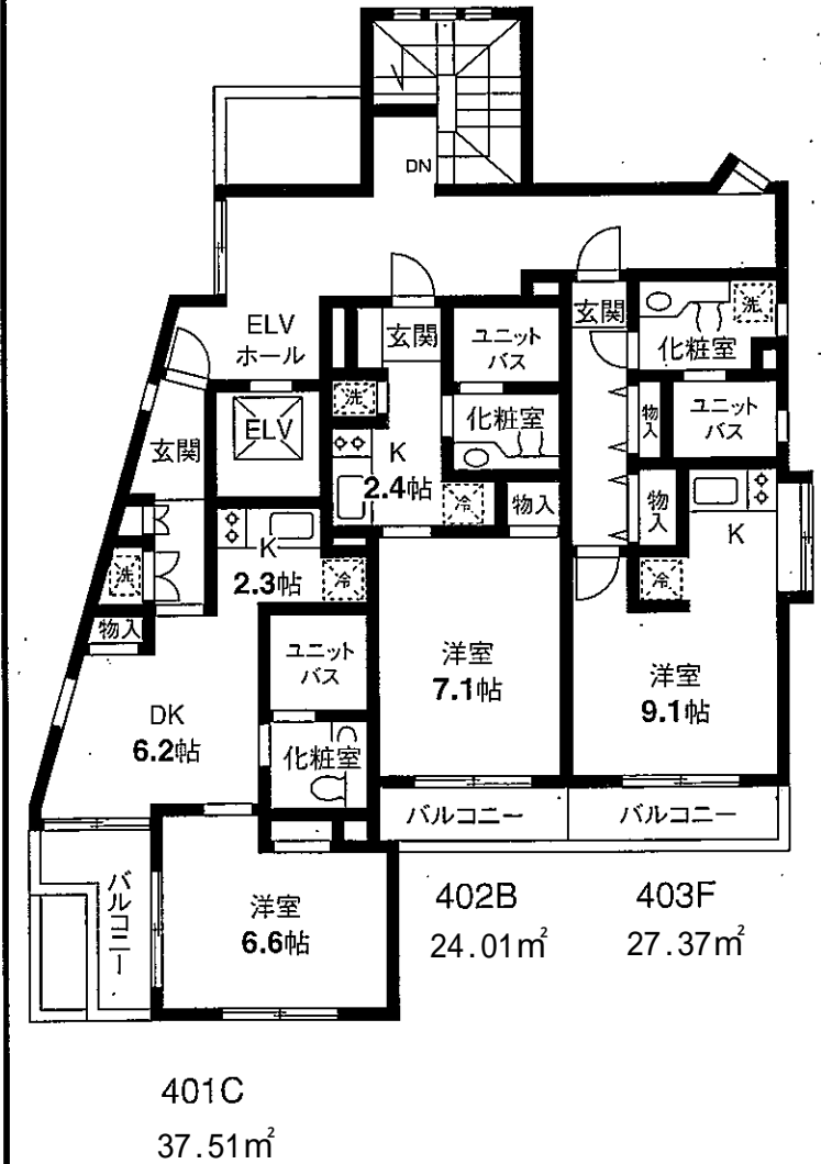
《4階平面図》
