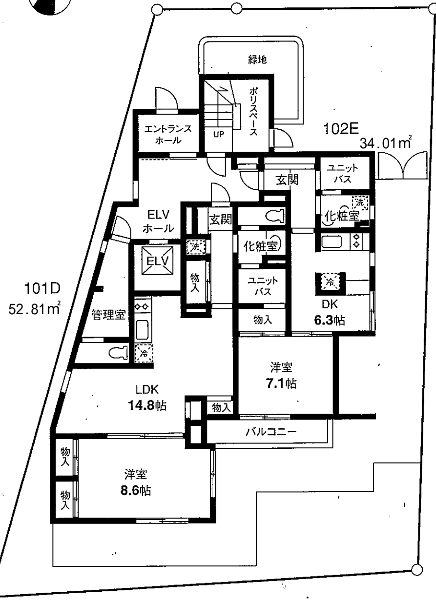
《配置図・1階平面図》
