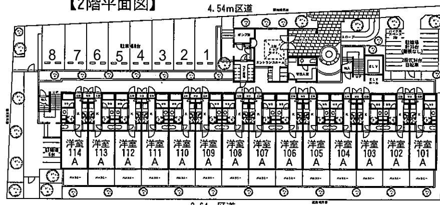
【配置及び1階平面図】
